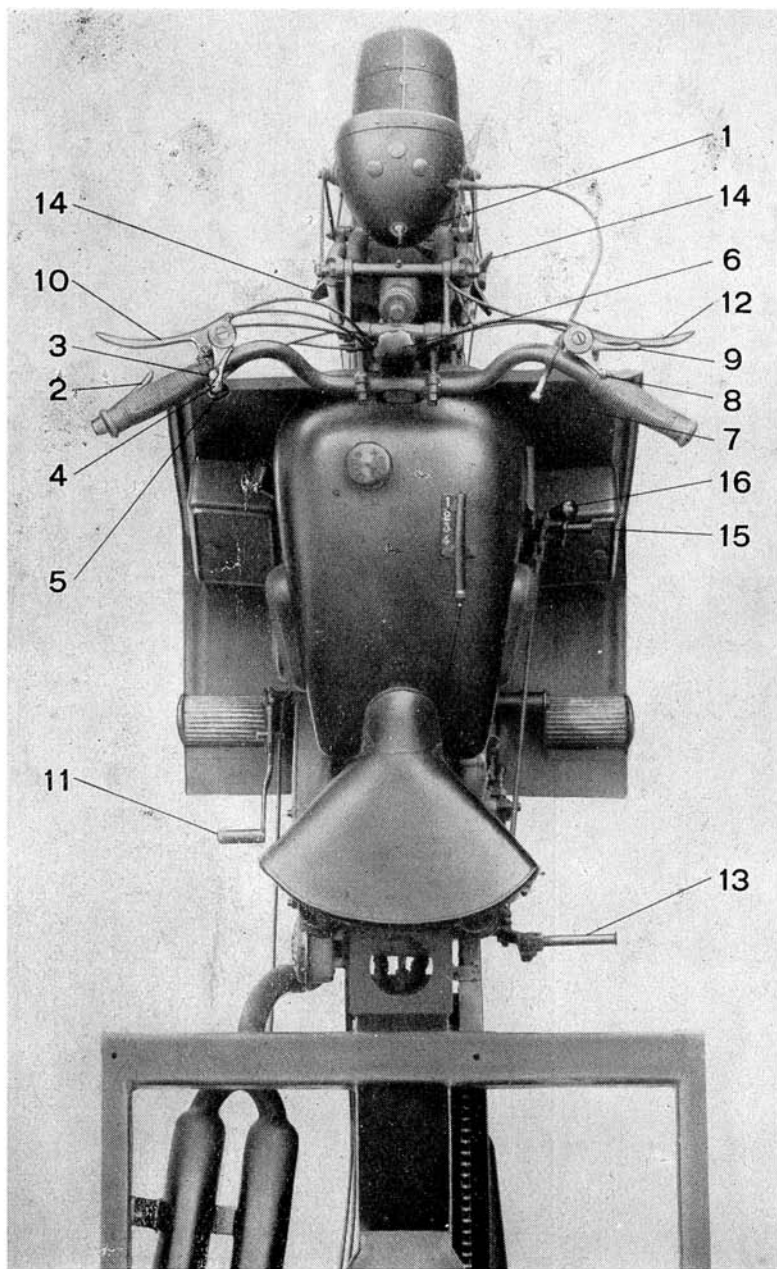
Fig. 5 Mototriciclo TRIALCE ( Comandi )
