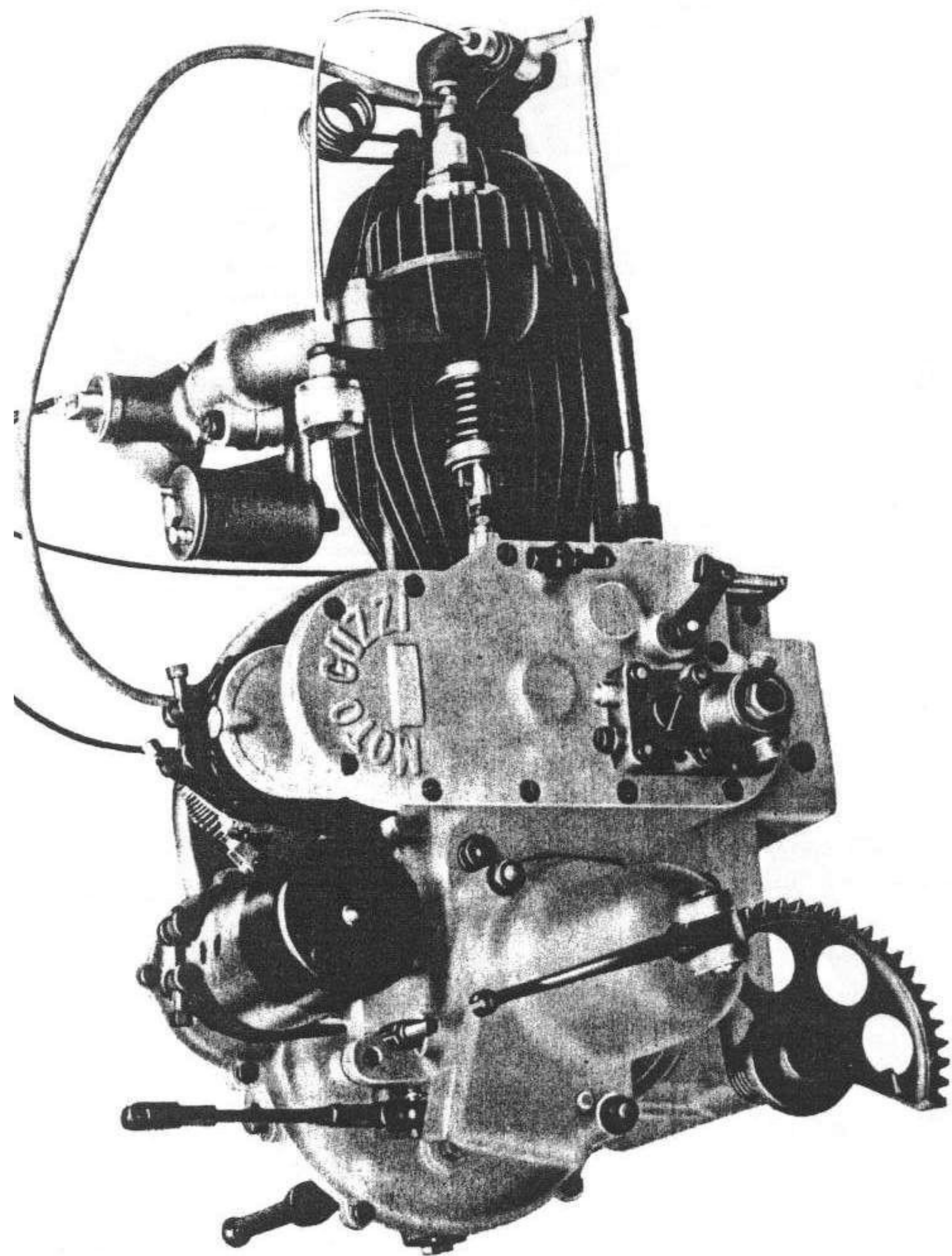
Fig. 1 - Gruppo motore cambio, lato distribuzione
