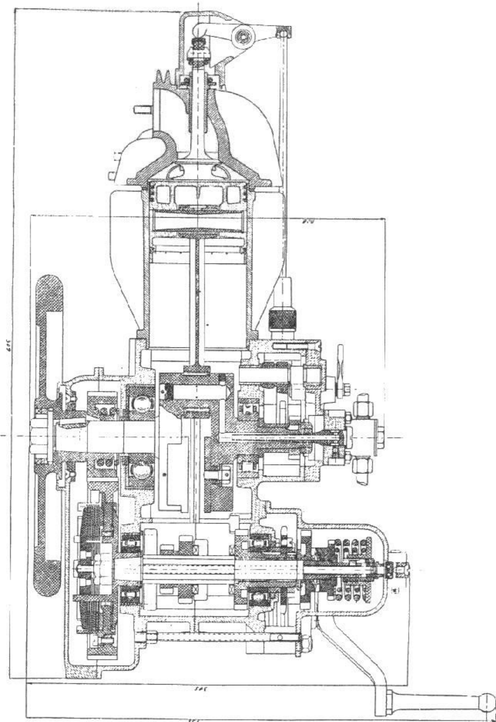
Sezione longitudinale orizzontale del motore.
