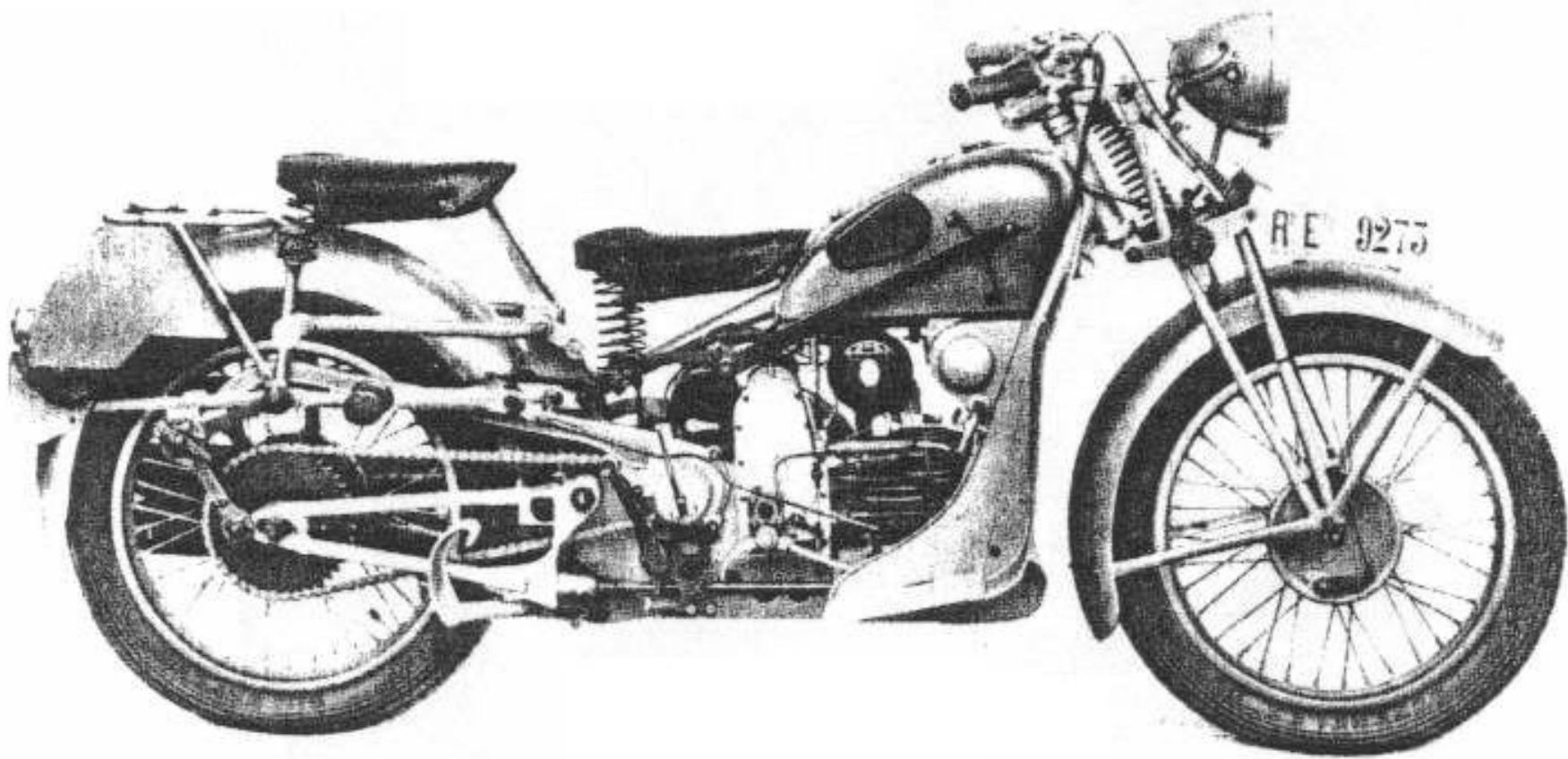
Fig. 12 - Moto "Biposto", lato distribuzione.
