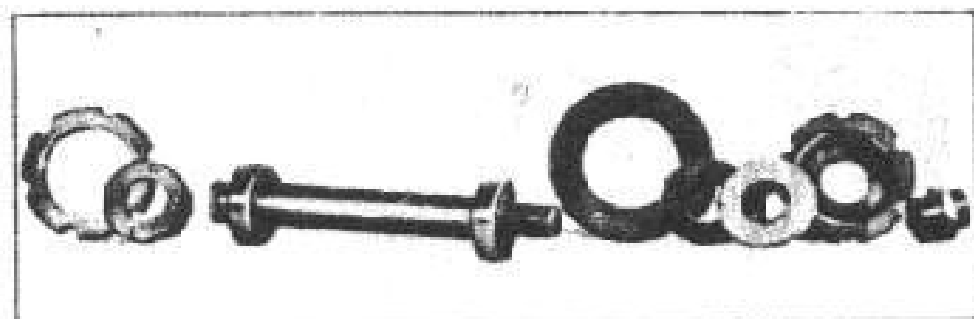
Fig. 88 - Mozzo posteriore. Ordine di montaggio dei vari pezzi.
