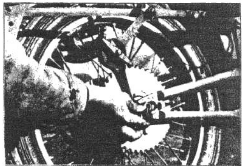
Fig. 20 - Come si leva la ruota posteriore - Il perno è già stato sfilato - Si vede nella mano il dado per perno forato.
