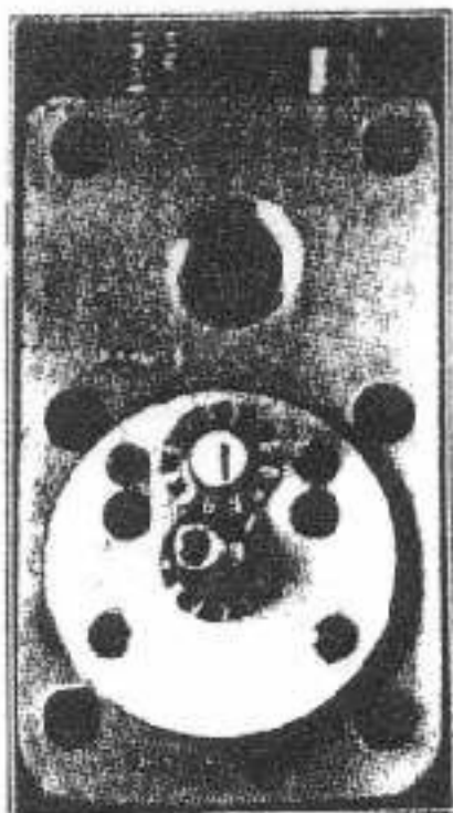
Fig. 71 - Il corpo pompa visto dall'interno. È visibile la pompa di mandata a ingranaggi.
