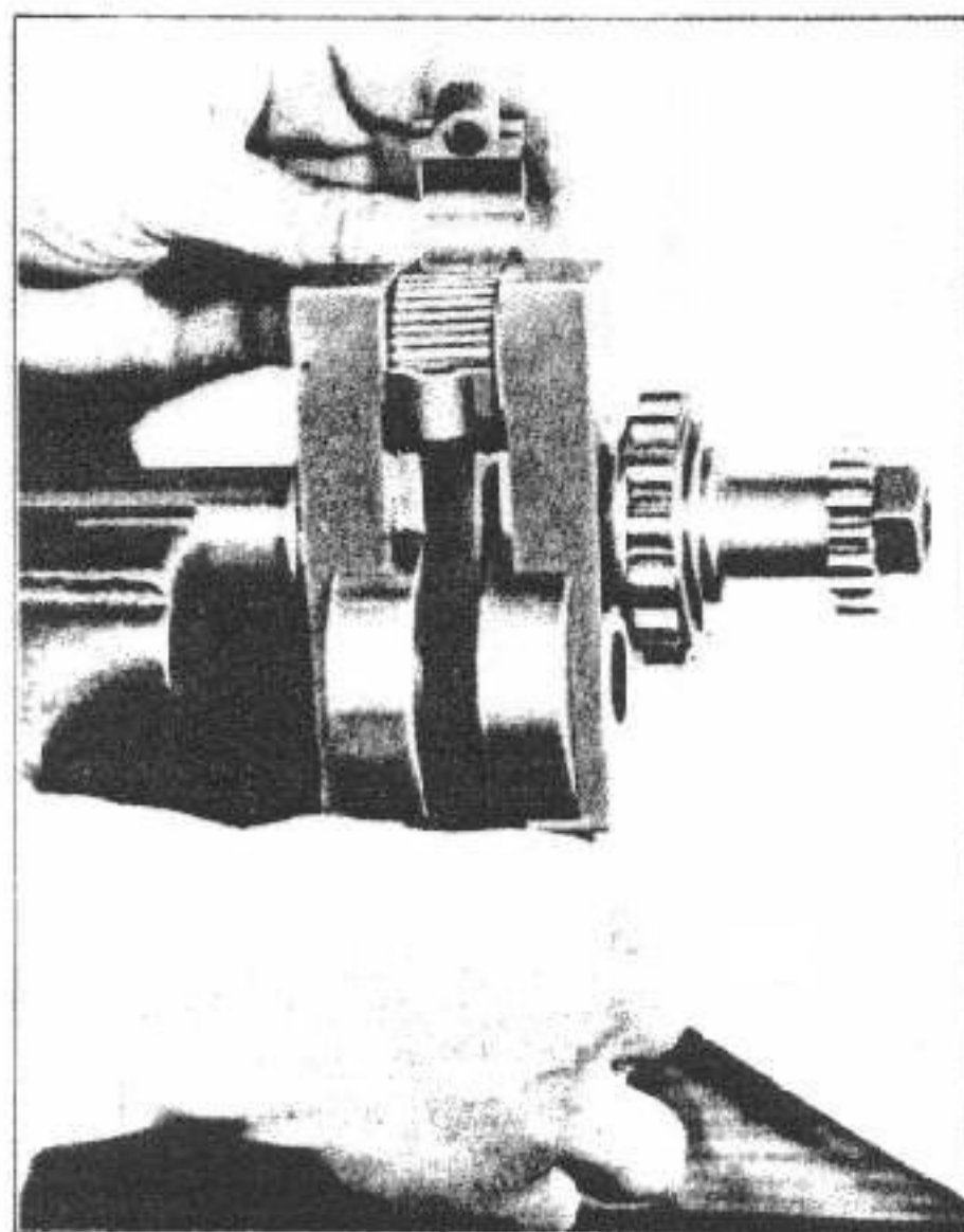
Fig. 59 - Come si montano i rullini della biella.
