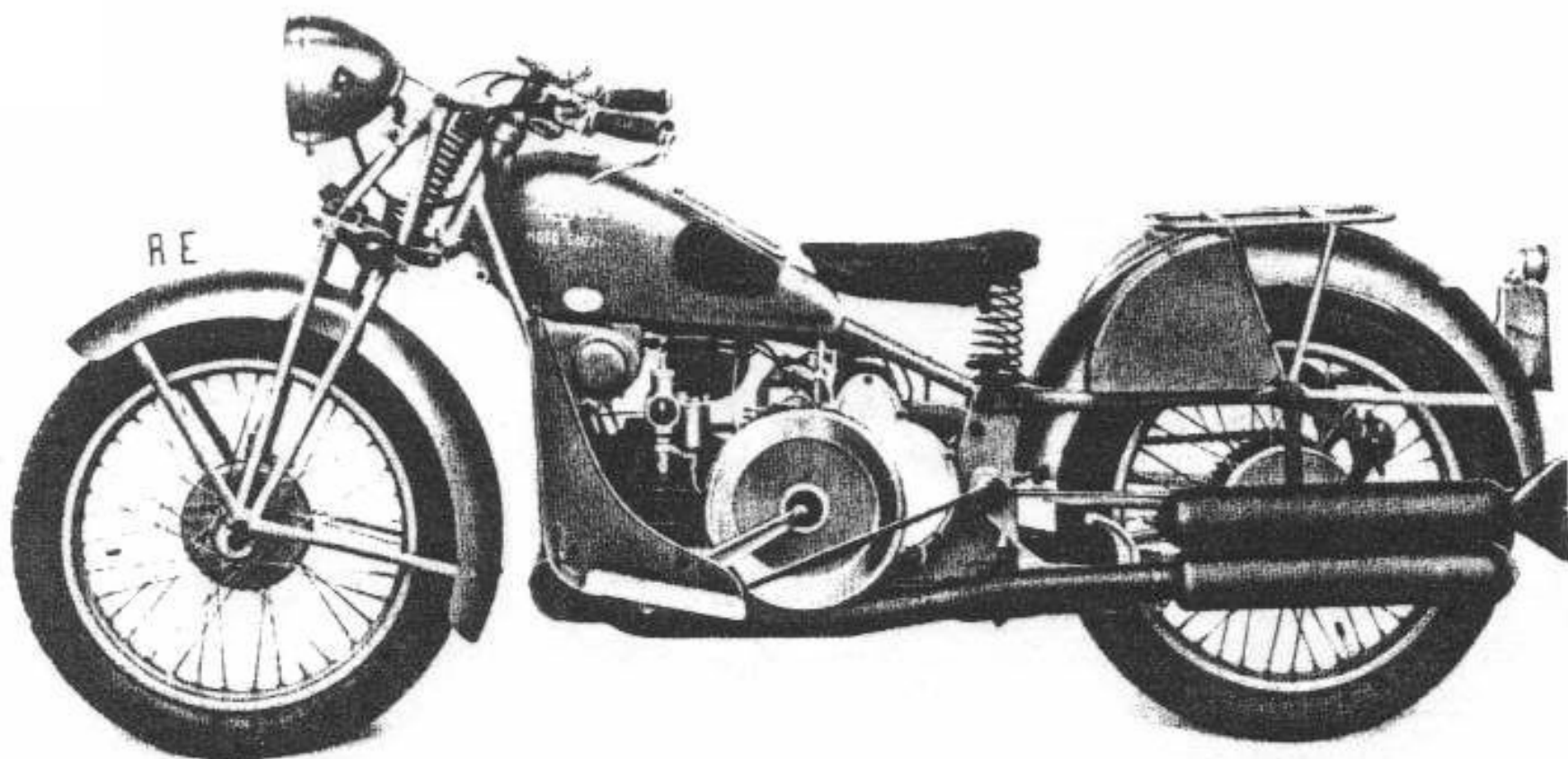
Fig. 7 - Moto "Monoposto" lato volano.
