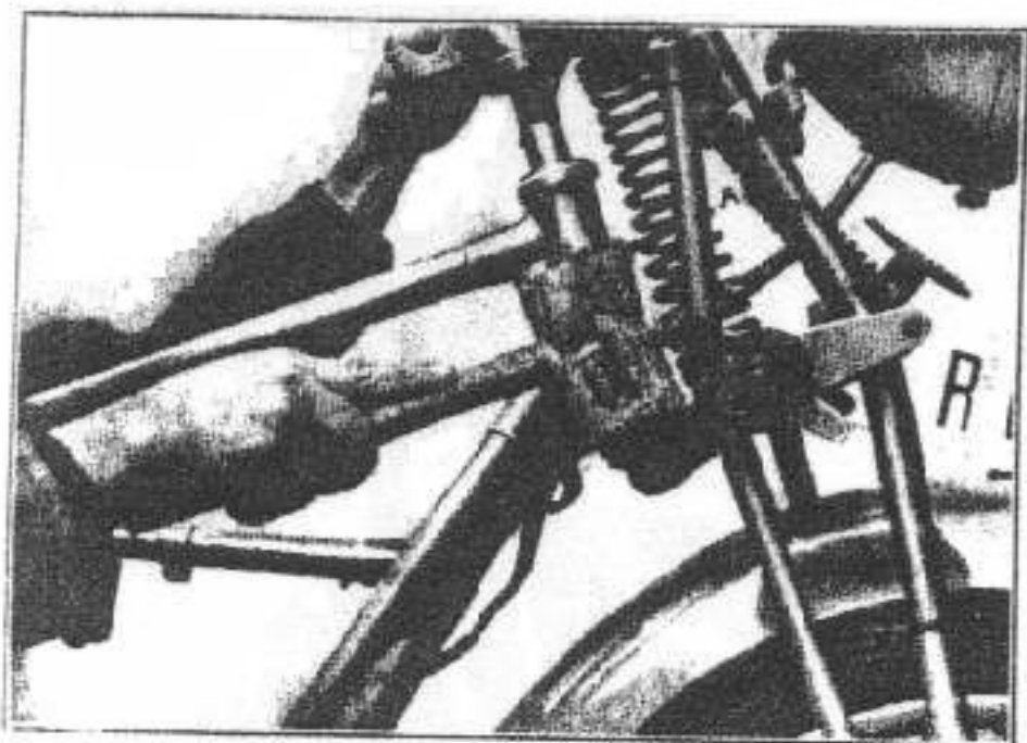
Fig. 29 - Come si sfilà il canotto di guida dalla testa di sterzo.
