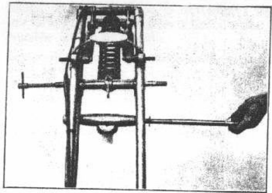
Fig. 35 - Come si levano i perni inferiori. Avvitare completamente e sfilare a sinistra.
