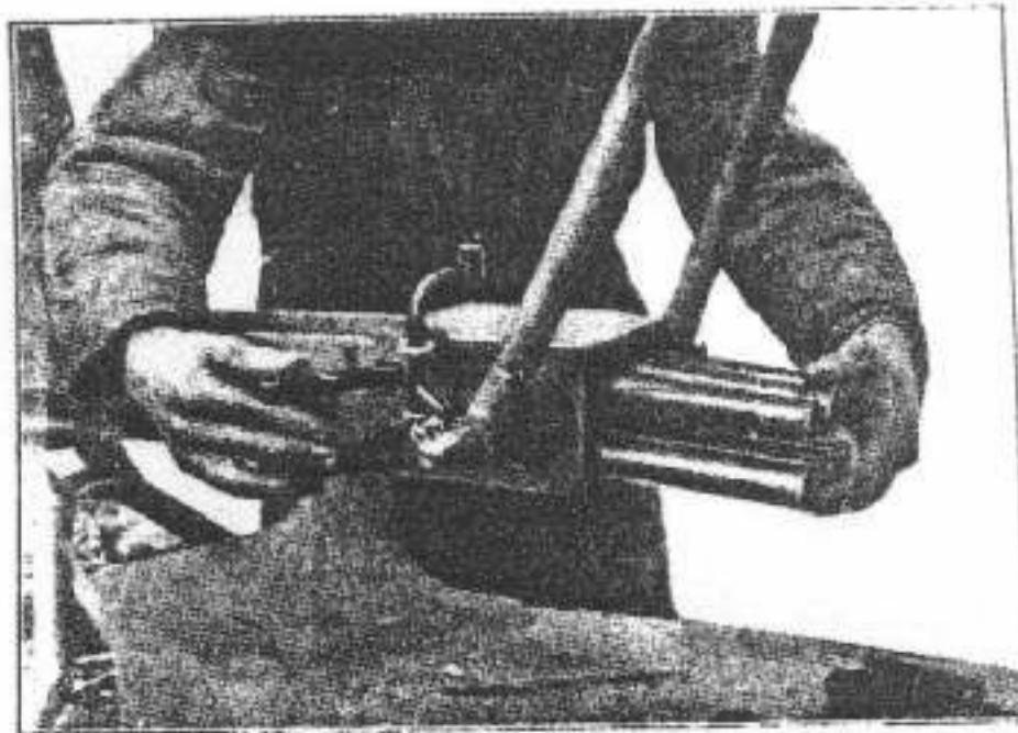
Fig. 27 - Come si levano le due cremagliere e il gruppo tubi reggi molla.
