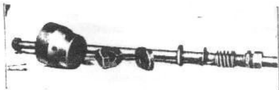
Fig. 86 - Da sinistra a destra: Uno dei 5 bulloncini, la scatola e i bloccetti maschio e femmina. Infilati nel tirante: la vanella di cuoio, il piattello, la molla e il morsetto di fissaggio.
