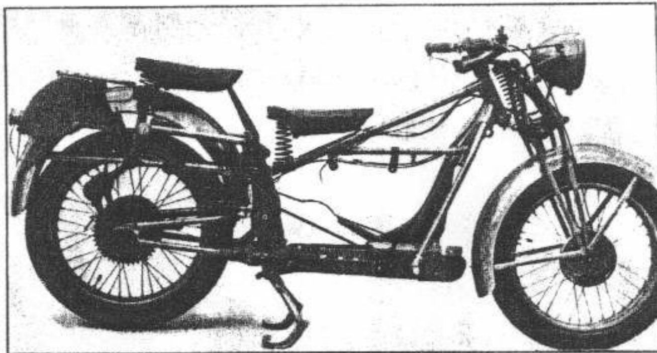
Fig. 5 - Telaio moto biposto visto dal lato destro.
