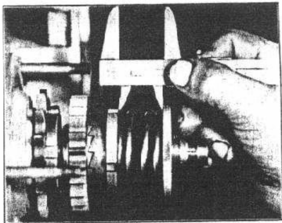
Fig. 62 - Come si regola la tensione delle molle della frizione. La misura normale, come indicato in figura, è mm. 28.
