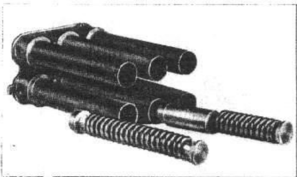
Fig. 84 - Moto biposto. Si notino lo spessore, la molla e la bussoletta di pressione laterali (a sinistra) e centrali.
