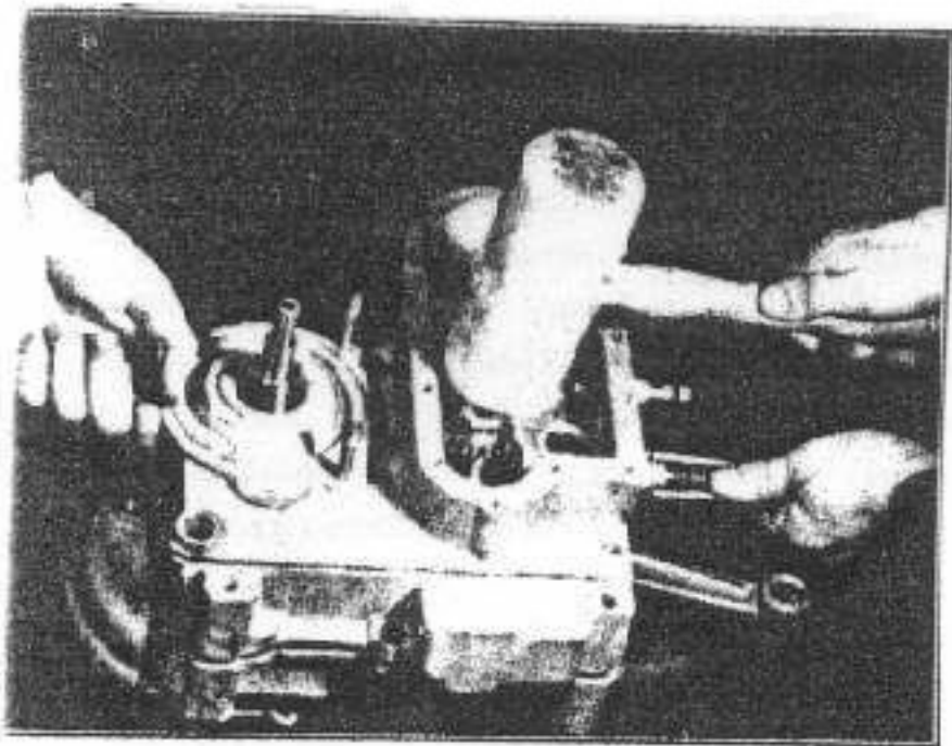
Fig. 46 - Come si apre il carter.
