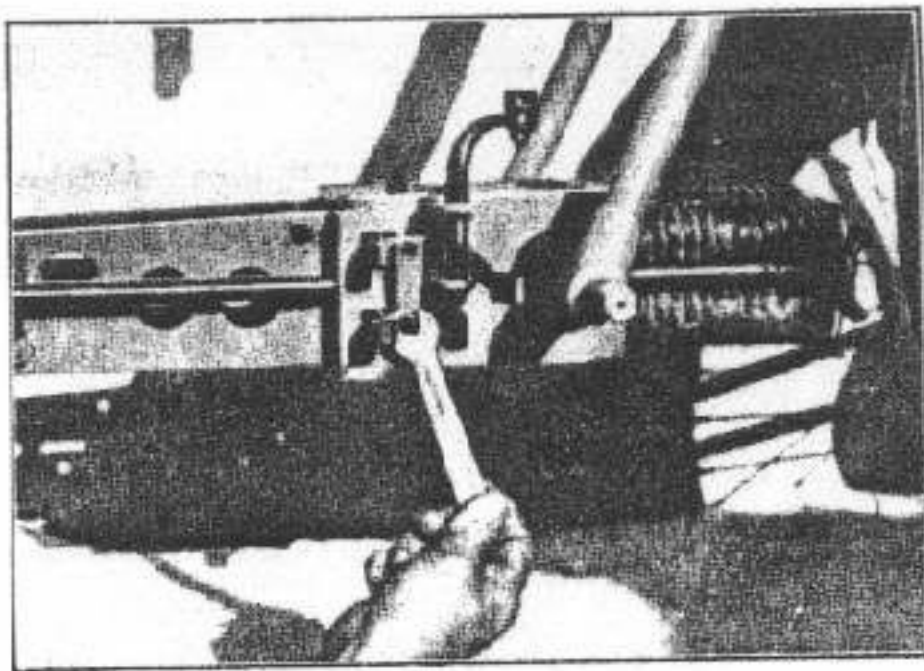
Fig. 25 - Come si leva la piastrina di fermo delle cremagliere.
