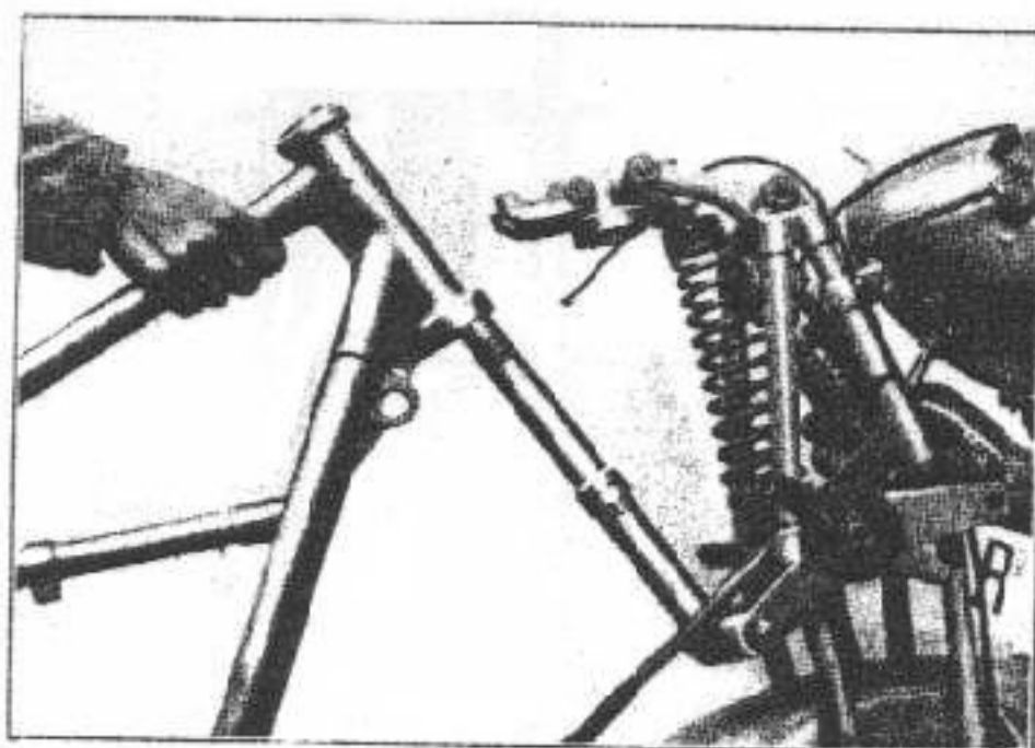
Fig. 30 - Come si sfilà il canotto di guida dal canotto del telaio (pipa di sterzo).
