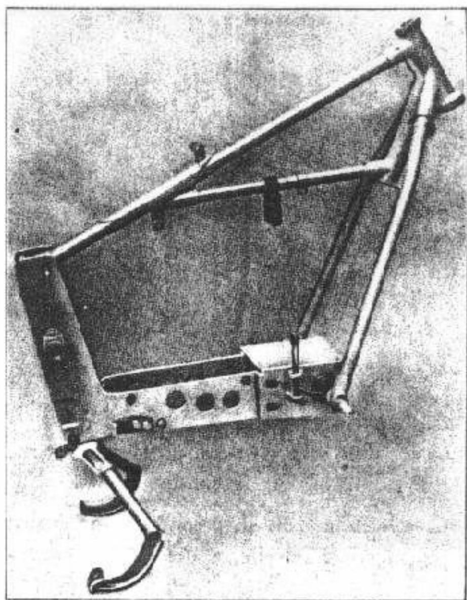
Fig. 31 - Vista del telaio centrale.
