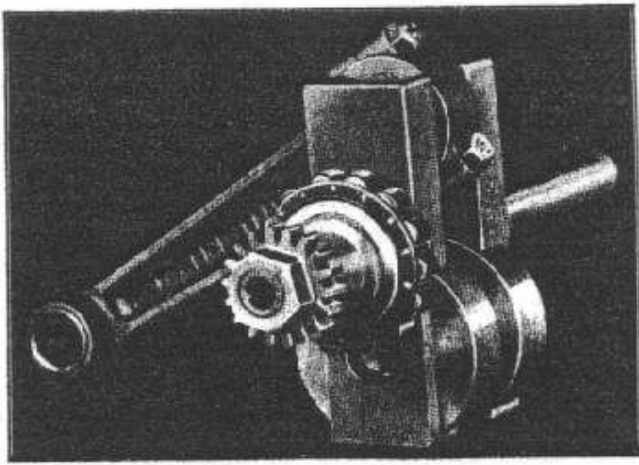
Fig. 56 - Gruppo albero a gomito biella visto dal lato distribuzione. Si notino il dado smussato all'esterno e la bulinatura di sicurezza.
