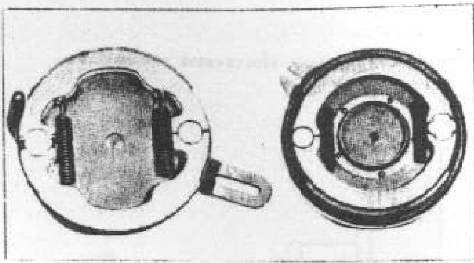
Fig. 89 - Piatto portaceppi posteriore e anteriore.
