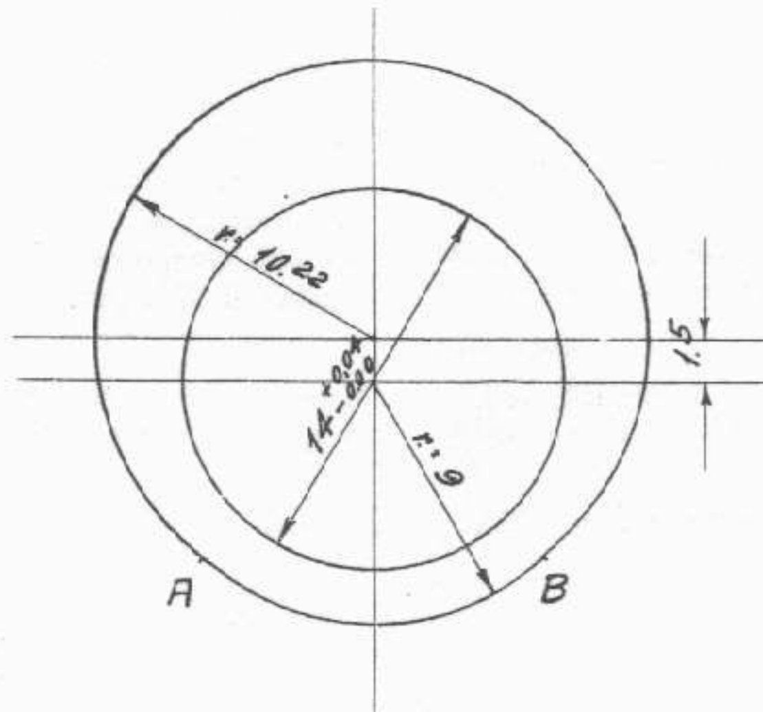
Fig. 73 - Schema sede delle palette.
