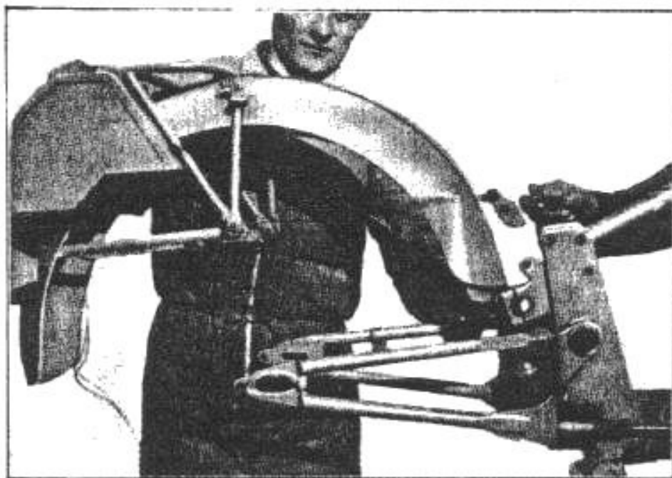
Fig. 19 - Come si leva il gruppo parafrango - Cassette Porta bagagli - Porta targa.
