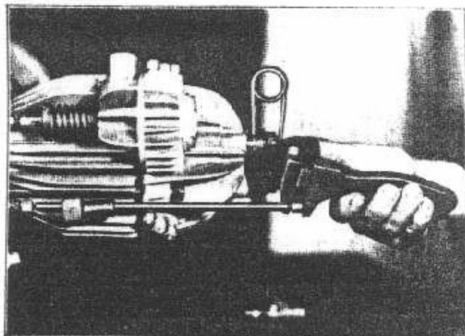
Fig. 76 - Come si monta l'asta di comando per bilanciere di scarico.
