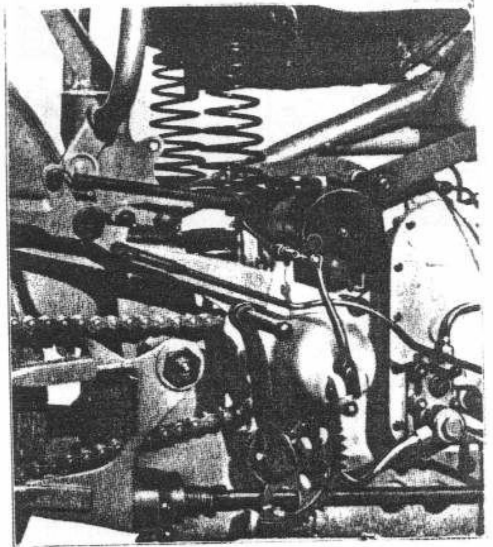
Fig. 10 - Moto biposto - Gruppo frizione - Avviamento Pompa olio.
