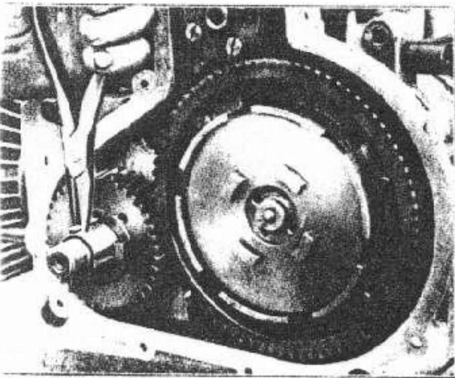
Fig. 41 - Levare la chiavella prima di sfilare il pignone motore.
