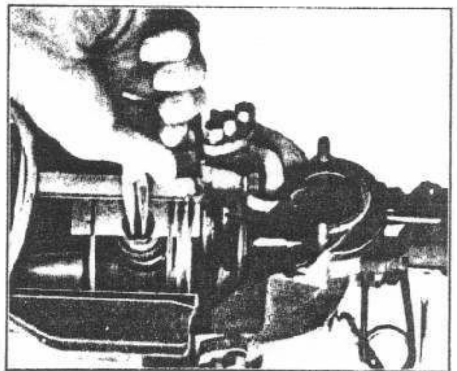
Fig. 39 - Come si leva la molletta (sinistra) che lassa lo spinotto. (Il motore è sezionato).
