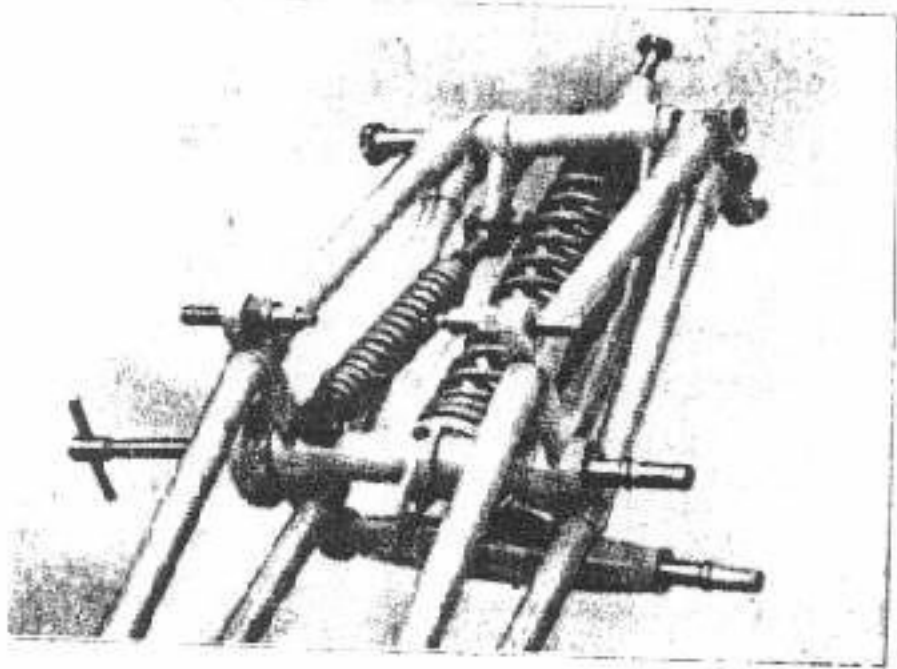
Fig. 34 - Come si levano i perni inferiori.
