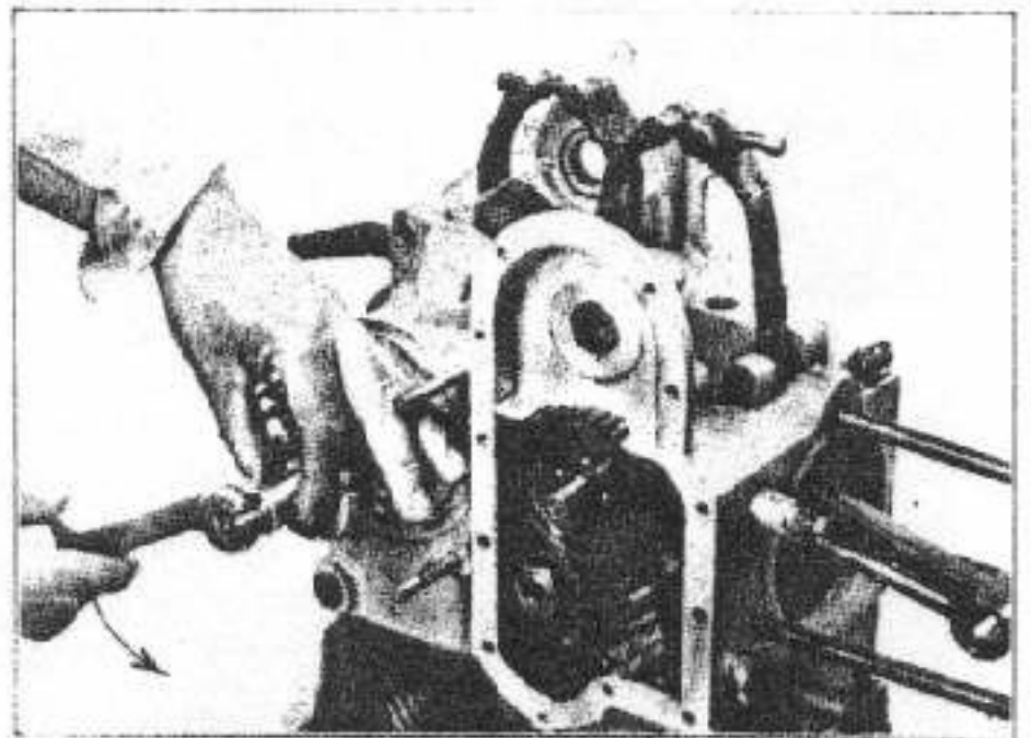
Fig. 42 - Come si leva l'asta interna di comando frizione.
