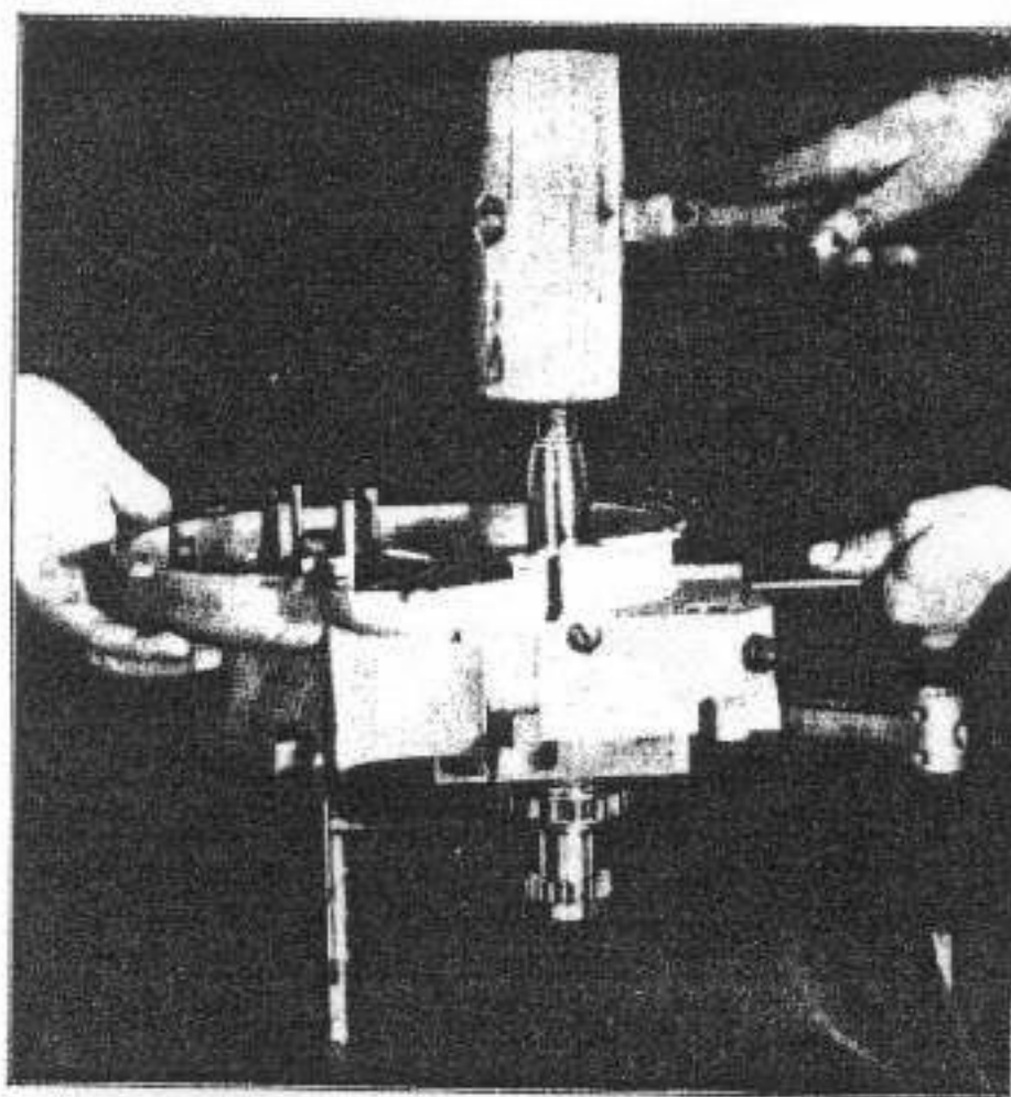
Fig. 48 - Come si leva il gruppo albero a gomito biella. Tenendolo sospeso il mezzo carter e battendo dall'esterno verso l'interno.
