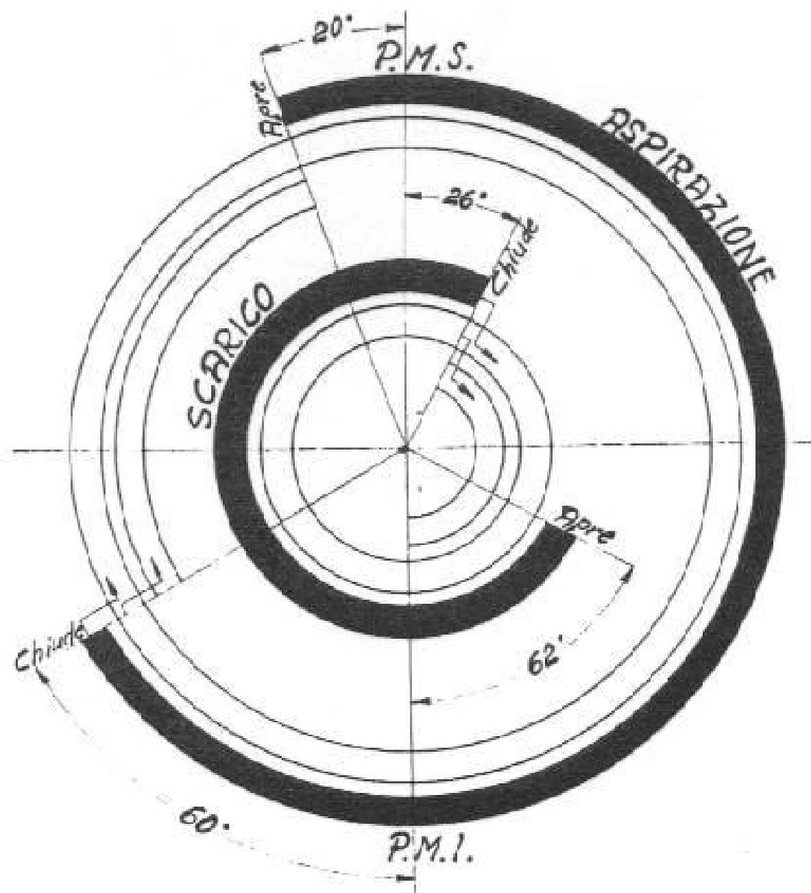
Diagramma angolare di distribuzione riferito all'asse motore
