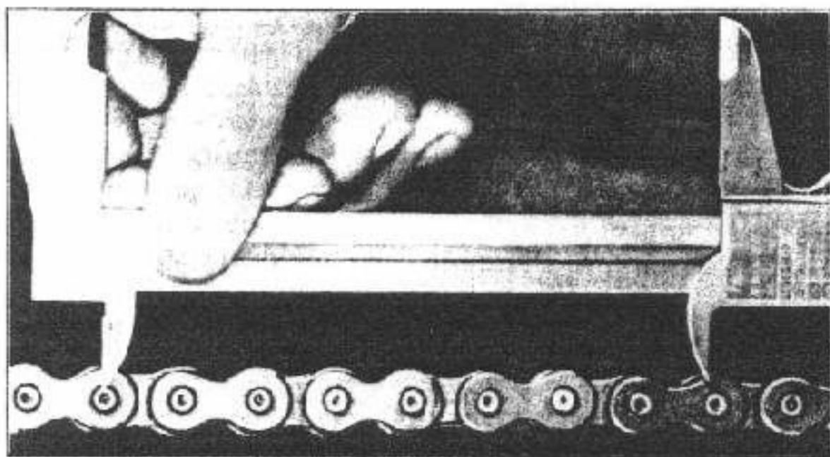
Fig. 56 - Come si controlla l'allungamento della catena di trasmissione.
