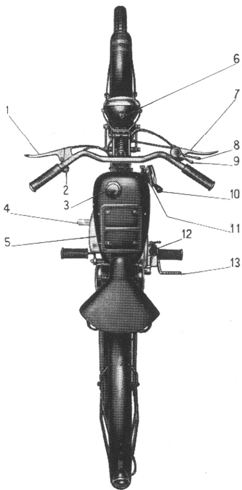
Fig. 3 - Motoleggera « 65 cm 3 » (comandi ed accessori)
