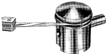
Fig. 23 - Controllo, mediante spessimetro a lame, del giuoco fra scanalatura pistone e fascia elastica
