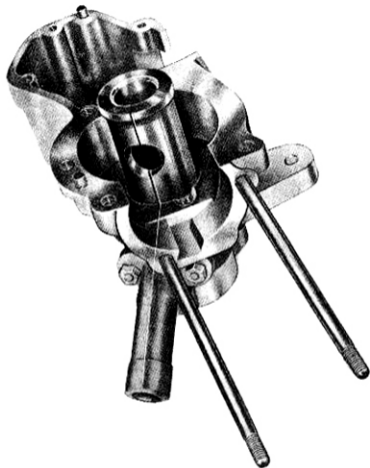
Fig. 27 - Linee di riferimento per la pressatura della boccia nel basamento sinistro
