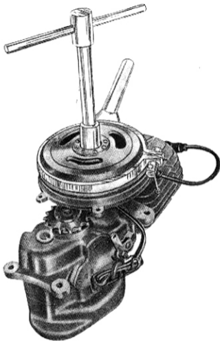
Fig. 15 - Come viene tolto il dado per volano magnetico
